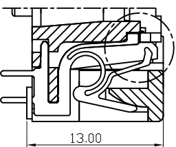
SEC.A-A
